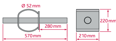
ADH 52 – Hochlastdorn
