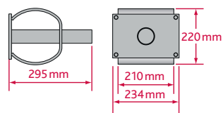
AHS 52 – Hochlast-Stahlhülse
