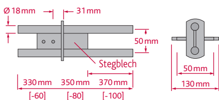
DSDS 50 – Doppelschubdorn
