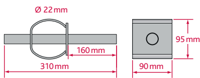
ADH 22 – Hochlastdorn
