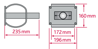
AHQ 35 – Hochlast-Stahlhülse mit Querweg ( \pm 16 mm)
