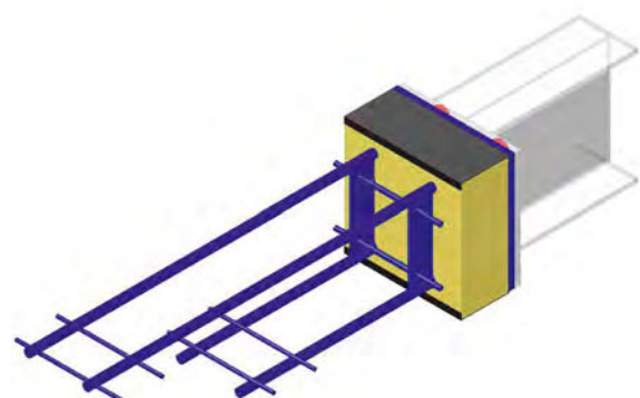
Stahlbauanschluss für Trägerprofile
