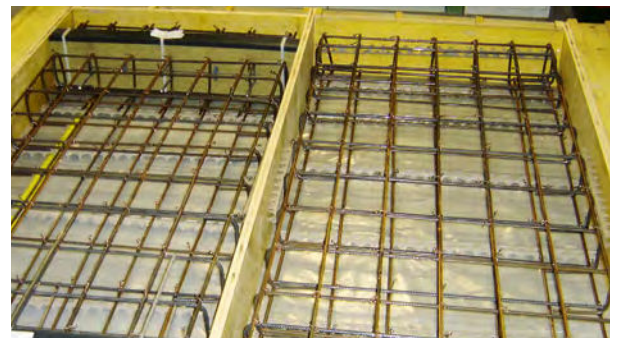
Bewehrung der Versuchsplatten: links mit ACINOX plus ® und rechts mit durchbetonierter Referenzplatte
