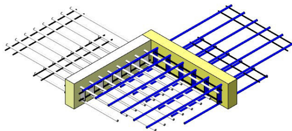
Zweiteilige Ecken für maximale Flexibilität
