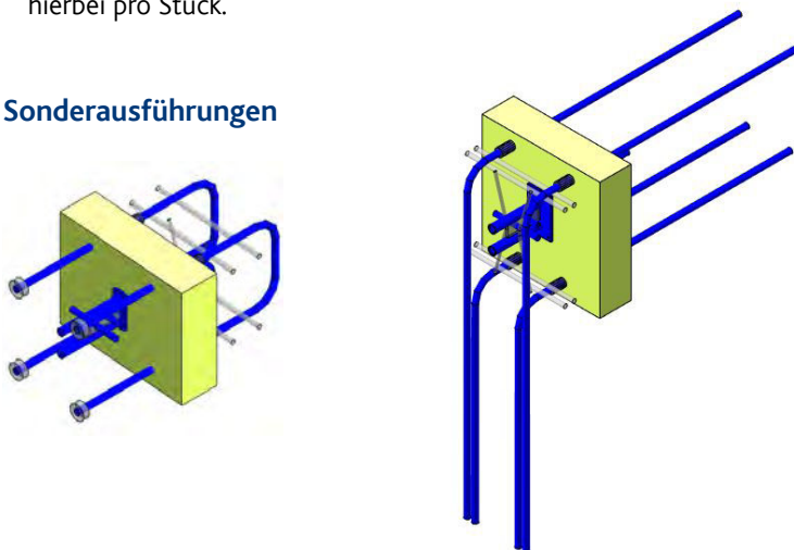
Mit kürzeren Anschlussstäben und Endverankerungen (Konsole in 2. Etappe)
