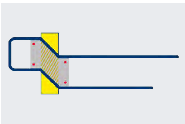
Bügelemente mit Versatz
