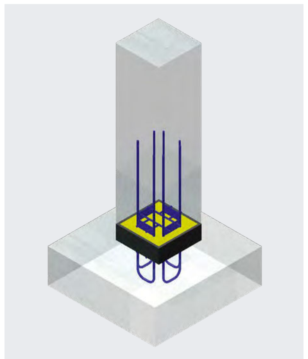
Stützenanschlüsse
