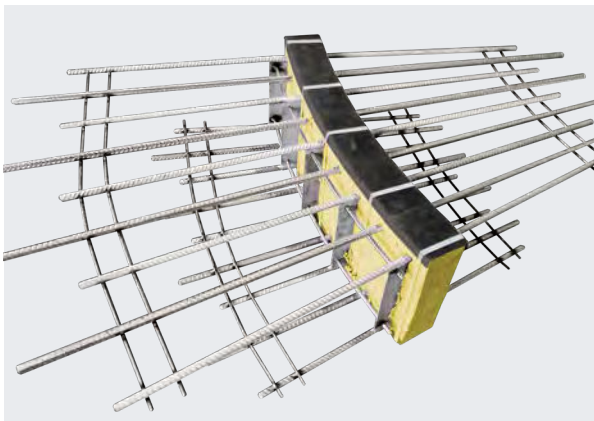
Radialelemente
