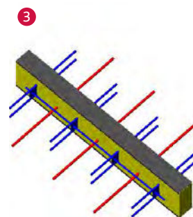
Querkräftanschluss mit Normalkraft z.B. QC-N+240
