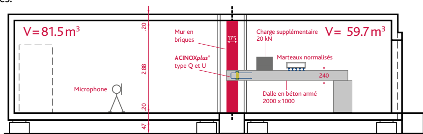
Configuration de la mesure phonique au laboratoire
