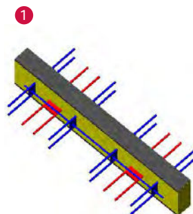
Elément d'effort tranchant avec raidisseurs horizontaux par ex. QC-S2+240
