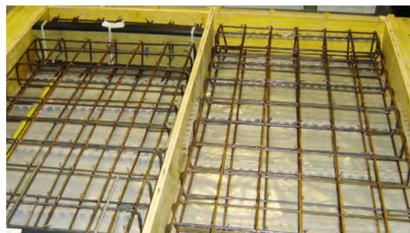
Armature des dalles d'essai: à gauche avec ACINOXplus® et droite avec dalle de référence raccordée sans console isolante
