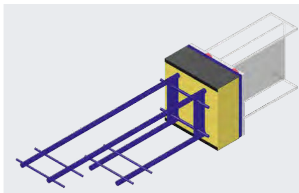
Raccordement d'une structure en acier à une structure en béton
