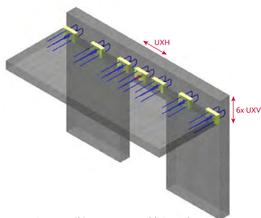
Exemple: marquise avec élément UXH+ additionnel disposé au milieu pour la rigidification horizontale
