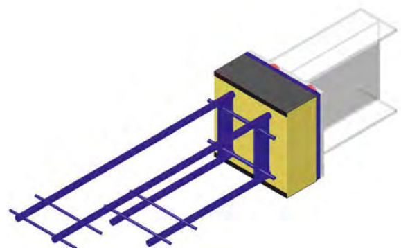
Raccordement d'une structure en acier à une structure en béton
