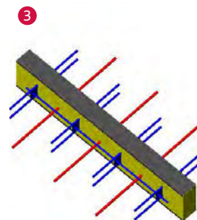
Elément d'effort tranchant avec effort normal par ex. QC-N+240
