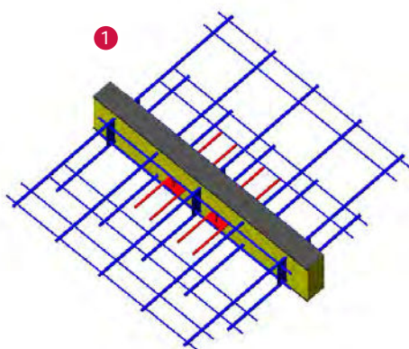
Console de flexion avec raidisseurs horizontaux par ex. KD-S2+240
