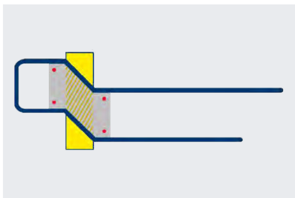
Eléments à étriers à hauteur décalée
