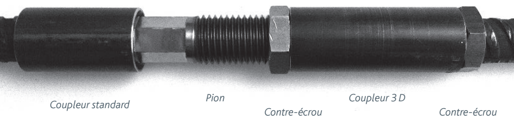
Contre-écrou
