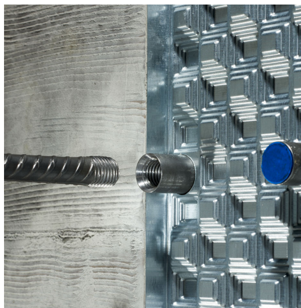
PYRABAR Typ PU, Bügeltyp Zweischnittig
