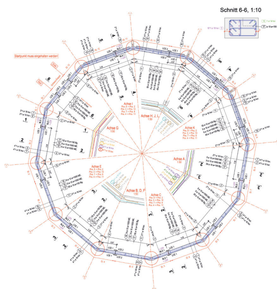
Geschlossener Bewehrungsring (Blau) des Zauberhutes.
