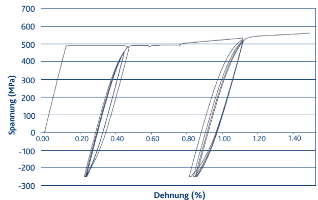
Spannungs-Dehnungs-Diagramm. Zyklische Erdbebensimulation gemäss ISO 15835-1-Versuchsanordnung
