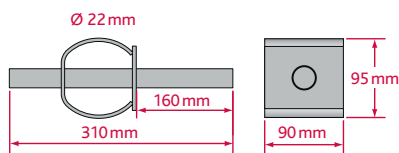
ADH 22 – Hochlastdorn
