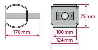
AHQ 18 – Hochlast-Stahlhülse mit Querweg (± 12 mm)
