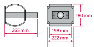
AHQ 42 – Hochlast-Stahlhülse mit Querweg (± 23 mm)
