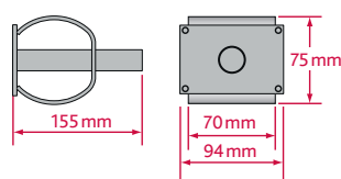
AHS 18 – Hochlast-Stahlhülse
