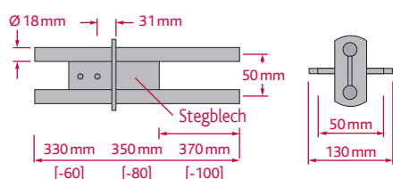
DSDS 50 – Doppelschubdorn
