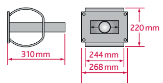
AHQ 52 – Hochlast-Stahlhülse mit Querweg (± 19 mm)
