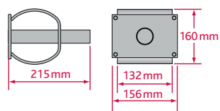
AHS 35 – Hochlast-Stahlhülse
