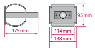
AHQ 22 – Hochlast-Stahlhülse mit Querweg (± 10 mm)
