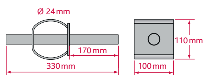
ADH 24 – Hochlastdorn
