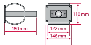
AHQ 24 – Hochlast-Stahlhülse mit Querweg (± 11 mm)
