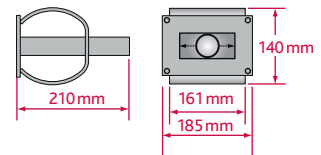
AHQ 30 – Hochlast-Stahlhülse mit Querweg (± 20 mm)
