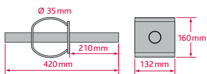
ADH 35 – Hochlastdorn
