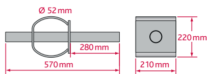
ADH 52 – Hochlastdorn
