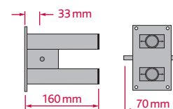
DSDSQ 50 – Stahlhülse mit Querschnitt (±12mm)
