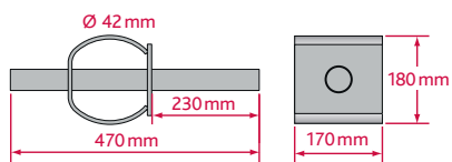
ADH 42 – Hochlastdorn
