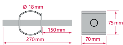
ADH 18 – Hochlastdorn
