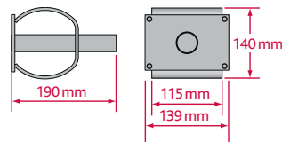
AHS 30 – Hochlast-Stahlhülse
