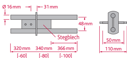
DSDS 30 – Doppelschubdorn
