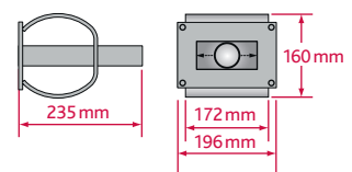
AHQ 35 – Hochlast-Stahlhülse mit Querweg (± 16 mm)
