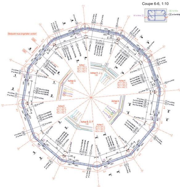
Vue en plan (anneau d'armature en bleu) : huit anneaux d'armature répartis en quatre lits reprennent les forces d'écartement du toit.
