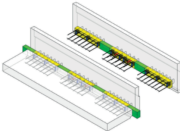
Regel-Detail der vorfabrizierten Fassadenbrüstung
