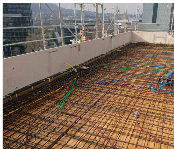
Ci-dessous : Consoles ACINOXplus® supportant les parapets
