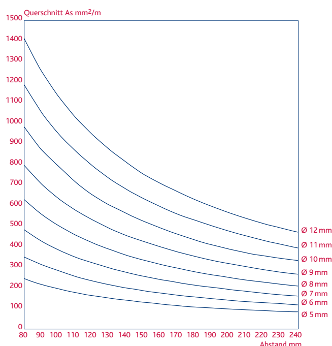
Grafische Abbildung von Querschnittsabstufungen
