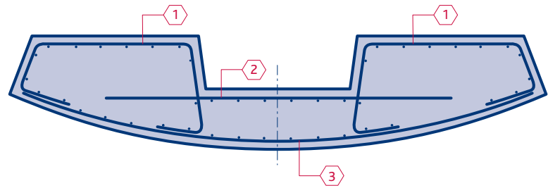
Beispiel: Vorfabrizierte Tübbing-Elemente
