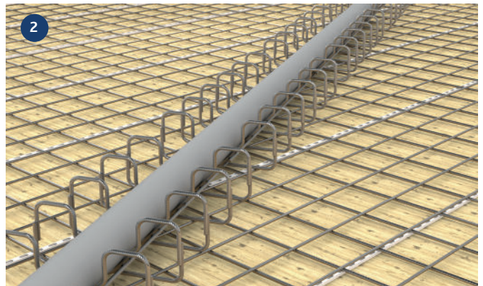
2 Leitung in die ersten Körbe einlegen. Halterungen bauseits anbringen.
