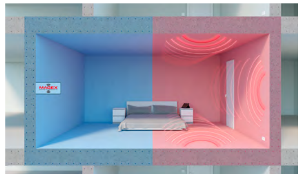
Magnetische Abstrahlung der Stahlbetonflächen bei entmagnetisierter (links) resp. nicht entmagnetisierter Bewehrung (rechts)
