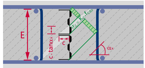
Abb. 13: Wirksame Höhe des Spannungsfelds
